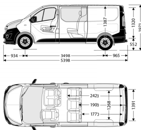
Furgon z podwójną kabiną Extra Long H1
