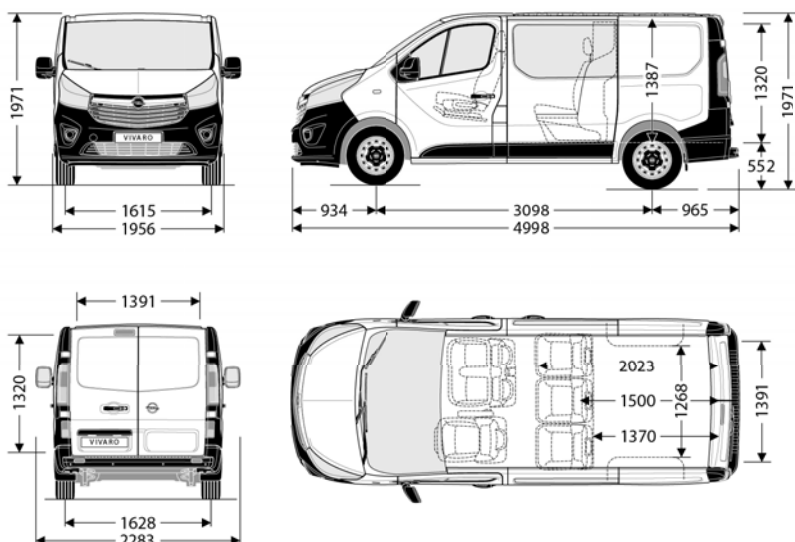
Furgon z podwójną kabiną Long H1
